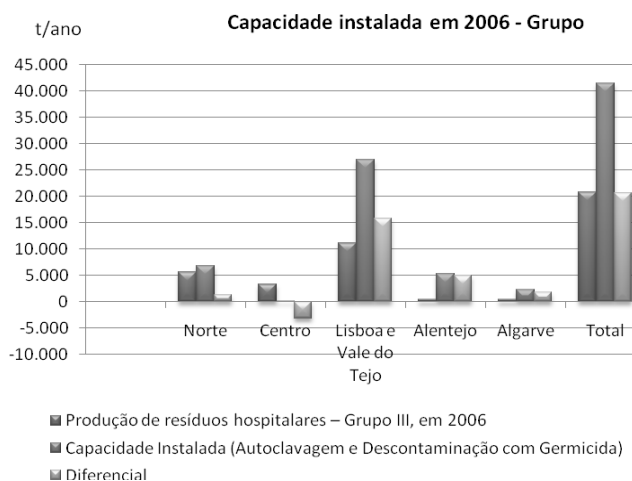
Figura 18 — Capacidade instalada para os resíduos do Grupo III e diferencial existente relativamente à produção estimada em 2006
